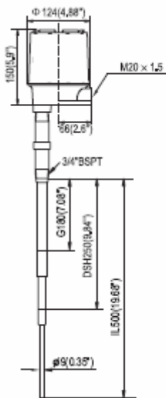
CT603-XXXX-168 外形图
