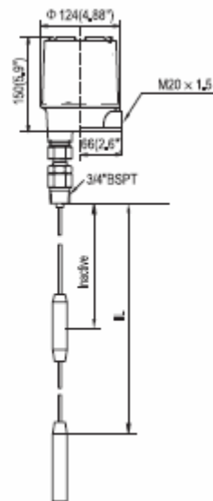
CT603-XXXX-179 外形图
