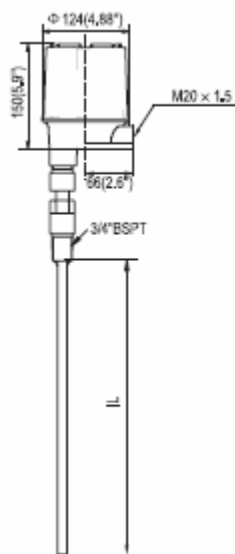
CT603-XXXX-174 外形图
