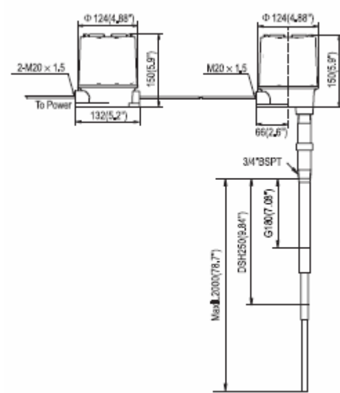
CT603-XXXX-XXX 分体式外形图
