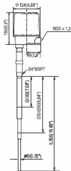
CT603-XXXX-169 外形图
