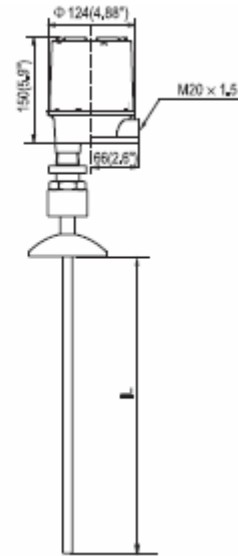
CT603-XXXX-183 外形图
