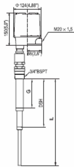
CT603-XXXX-182 外形图
