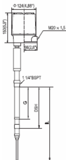
CT603-XXXX-172 外形图
