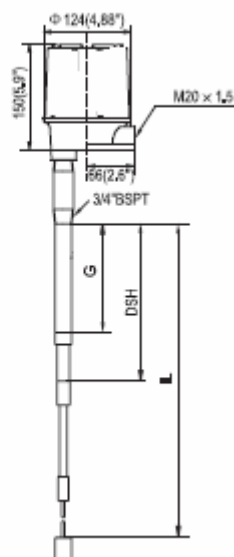
CT603-XXXX-173 外形图
