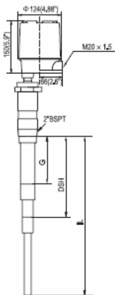
CT603-XXXX-170 外形图
