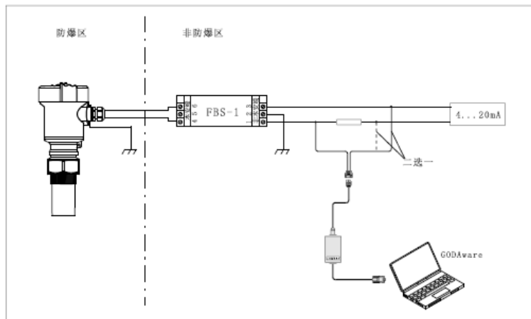
采用 GODAware 调试物位计
